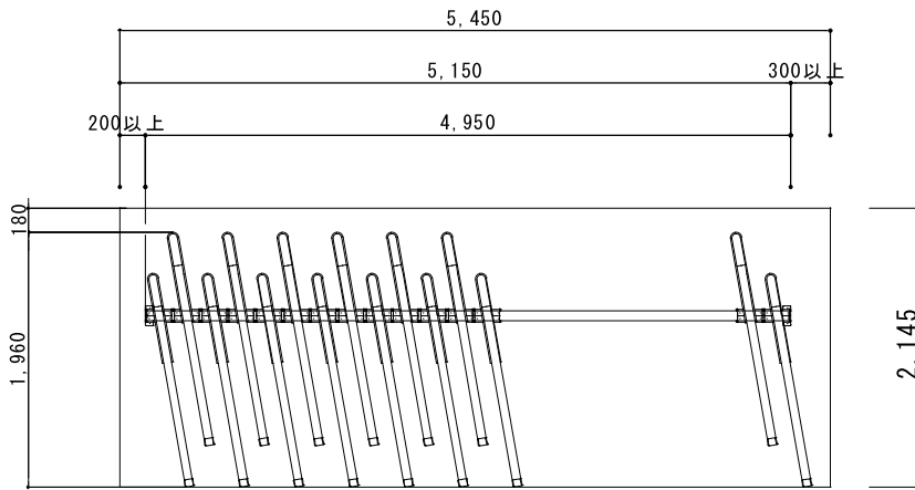
上段平面配置図 S=1/50
