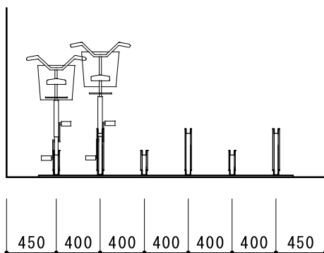
■ 正面図 S=1/50
