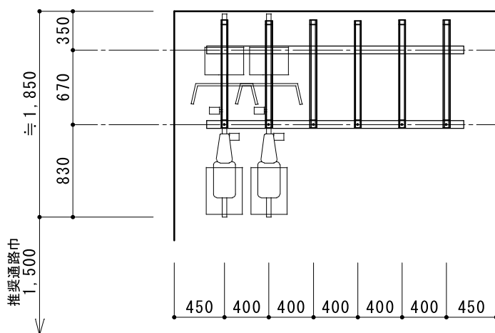
■ 平面図 S=1/50
