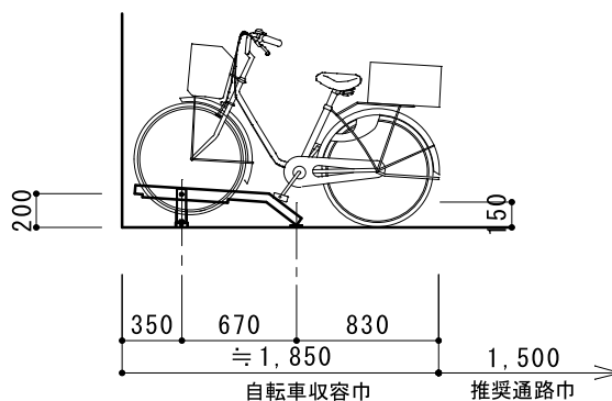
■ Lタイプ側面図 S=1/50
