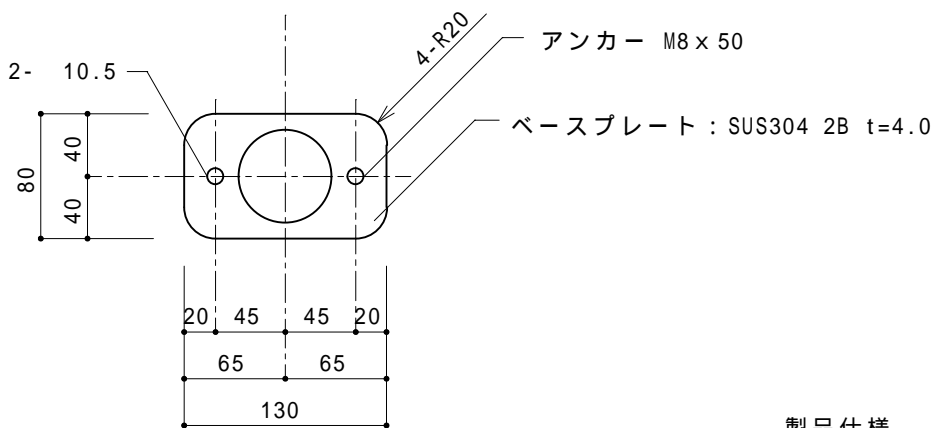
柱脚詳細図 S=1/5
