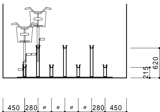
正面図 S=1/50
