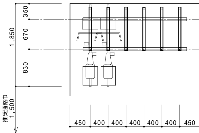
平面図 S=1/50
