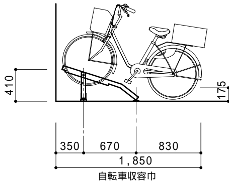
Hタイプ側面図 S=1/50
