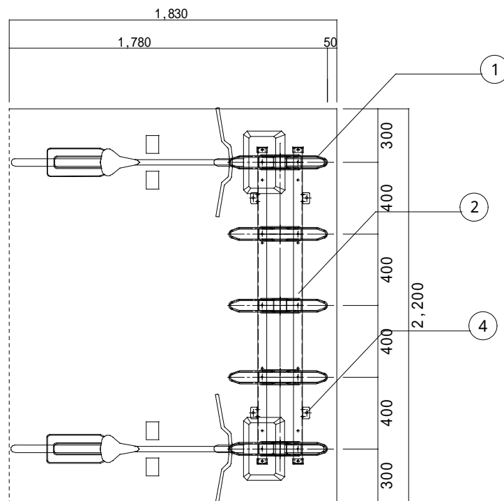
単列平面詳細図 1/30
