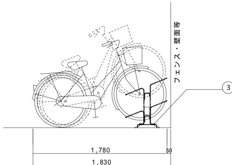
単列側面図 1/30
